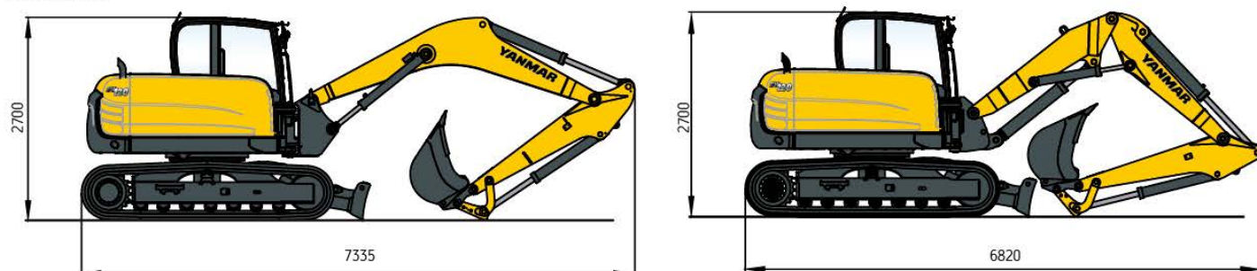
Abb. 2: Transportstellung
